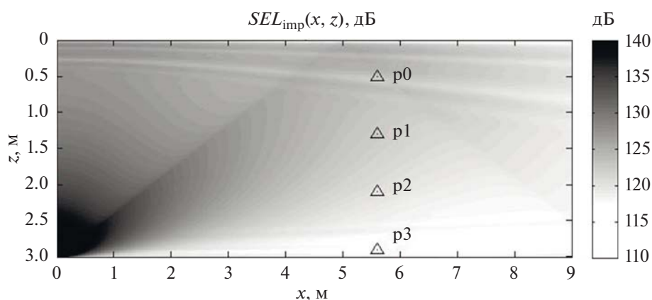
Рис. 9. Поле значений уровня энергии SEL_{imp}(x, z) распространяющегося акустического импульса, иллюстрирующее интерференцию прямых водных лучей с отраженными от дна и поверхности моря. Эквивалентный раку точечный источник расположен в точке x = 0 м, z = 2.99 м. Угол между осью z и проявляющейся линией соответствует критическому углу падения \theta_{cr} = 58.5^\circ .
