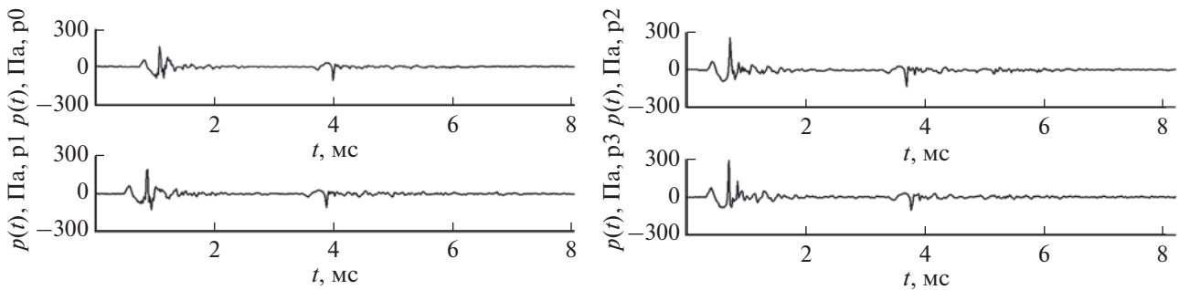
Рис. 6. Прямые и отраженные от морской поверхности акустические импульсы рака-шелкуна, измеренные 4-мя гидрофонами в горизонтальной плоскости (см. рис. 5б), излученные под небольшим углом к дну.
