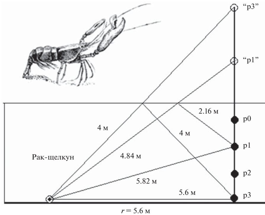
Рис. 5. Геометрическая схема для оценки радиуса r , на котором мог находиться рак-шелкун, излучивший акустический импульс, показанный на рис. 4а.
