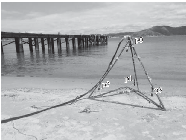
Рис. 2. Металлическая пирамида с установленными 4-мя измерительными гидрофонами.
