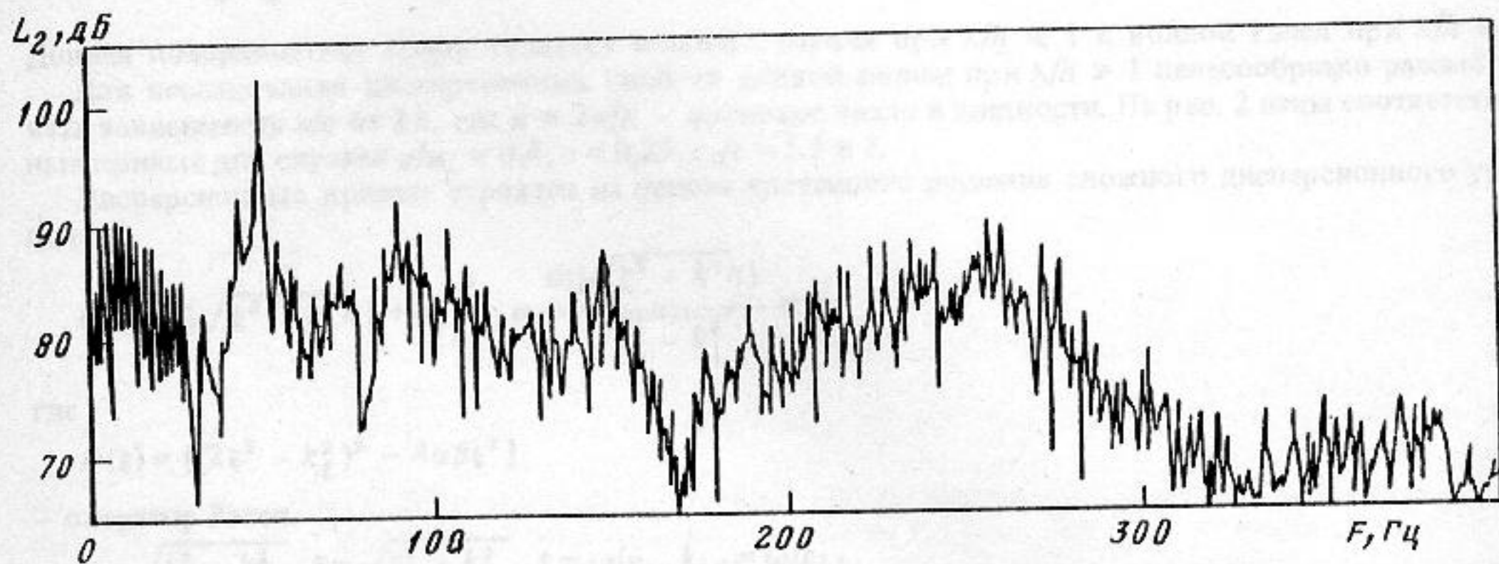
Рис. 3. Спектральная характеристика прошедшего через слой пены звукового потока
