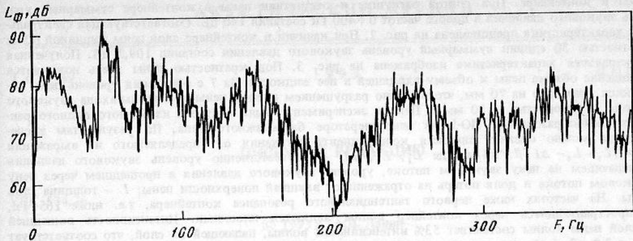
Рис. 1. Спектральная характеристика фонового звукового потока
