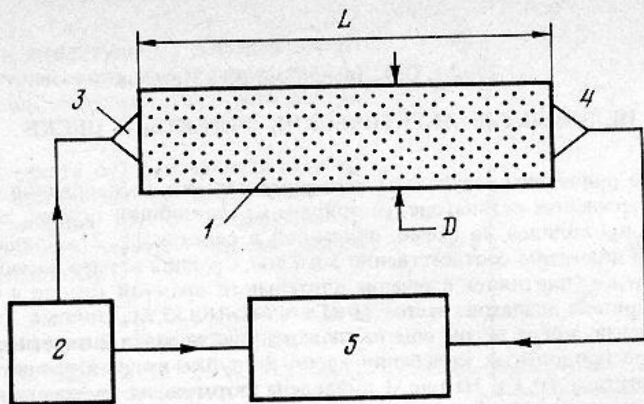
Установка для измерения времени пробега ультразвукового импульса в образце. 1 – образец; 2 – генератор импульсов напряжения; 3, 4 – излучатель и приемник ультразвуковых колебаний; 5 – измеритель временных интервалов
