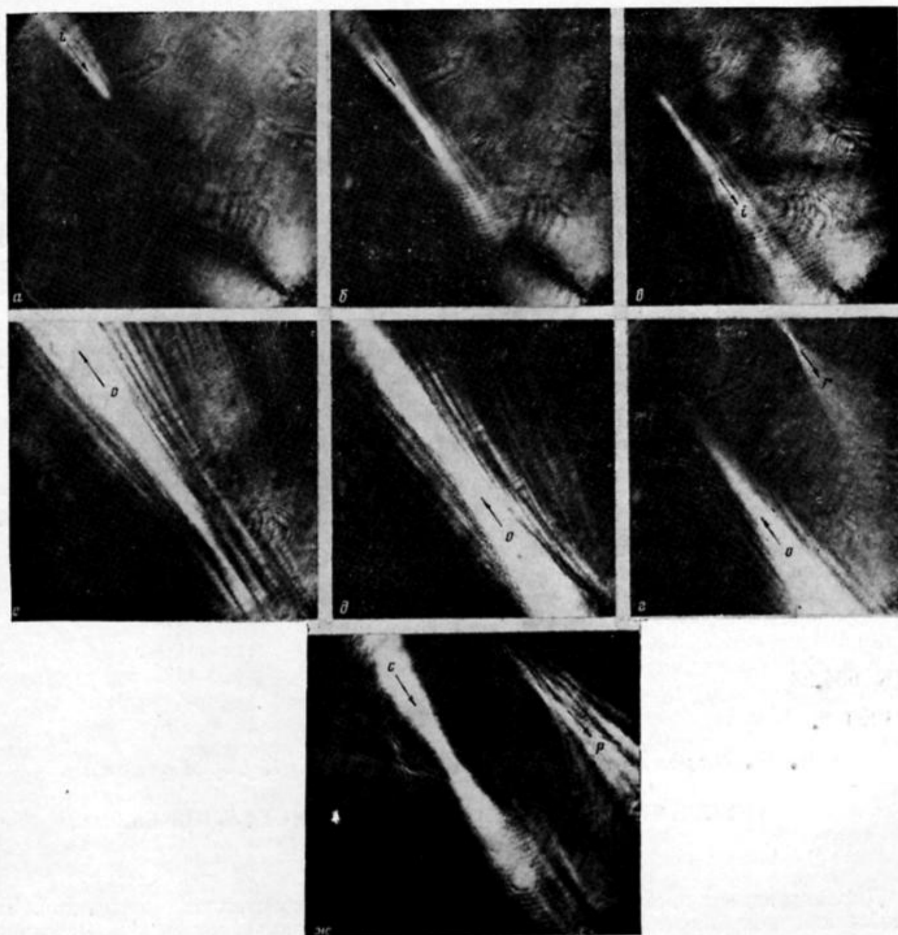
Рис. 2. Изображения распределений поля ультразвуковых импульсов в различных стадиях прохождения через акустический фокус. a, g — схождение в область фокуса, b, d — прохождение через область фокуса, e, e — выход из области фокуса. i — исходная волна, r — отражения исходного импульса в звукопроводе, o — обратная волна, p — отражение необращенных компонент обратной волны, c — «очищенная» обращенная волна
