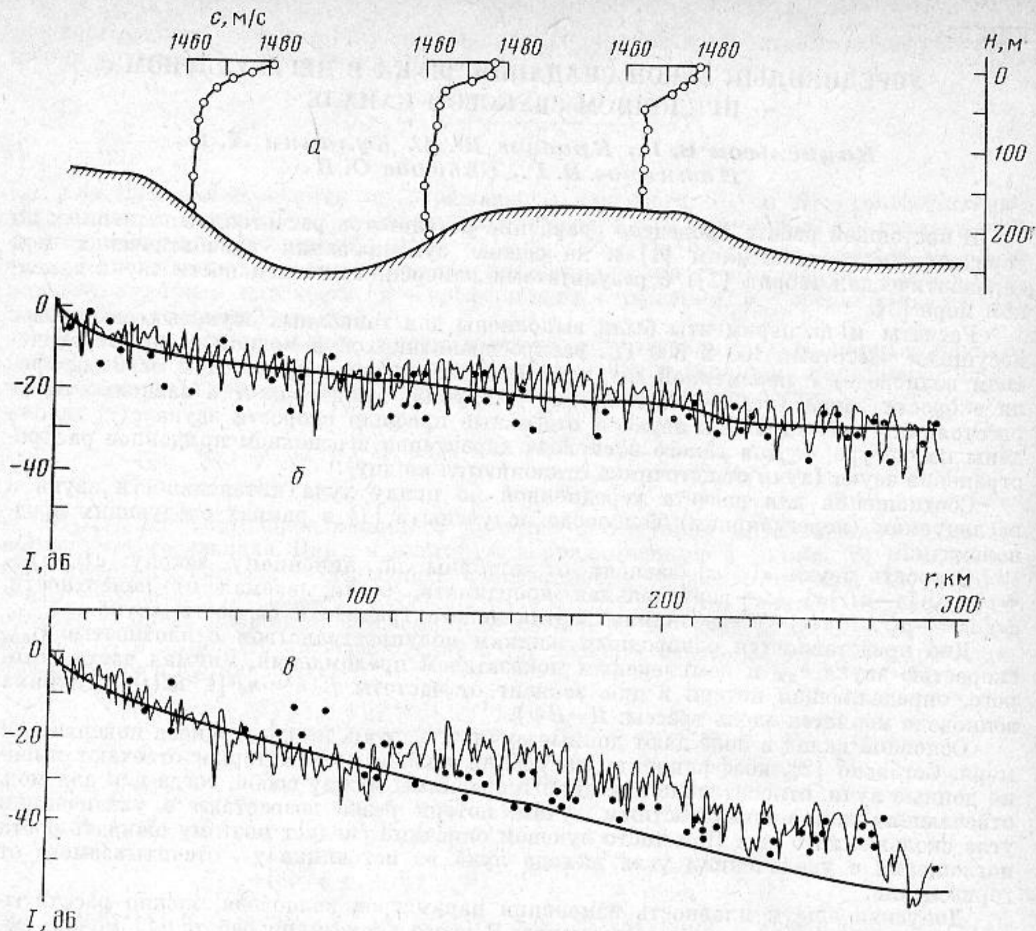
График зависимости нормированной интенсивности звука в волноводе от расстояния r ( I_1 = 10 \lg I/I_0 + 10 \lg r/r_0 , I_0 — интенсивность звука на расстоянии r_0 ): а — частота сигнала 300 Гц, б — зависимость глубины волновода H от расстояния r и отдельные профили скорости звука c вдоль волновода, в — частота сигнала 100 Гц
