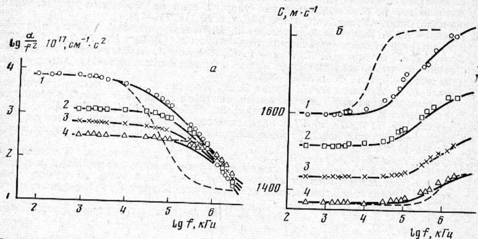
Зависимости поглощения (а) и скорости звука (б) от частоты для трансформаторного масла при температурах -20^\circ\text{C} (1), 0^\circ\text{C} (2), 20^\circ\text{C} (3) и 40^\circ\text{C} (4). Сплошные кривые — расчет по формуле (2), пунктирные — по формуле (1) при -20 и 40^\circ\text{C} ; точки — результат эксперимента
