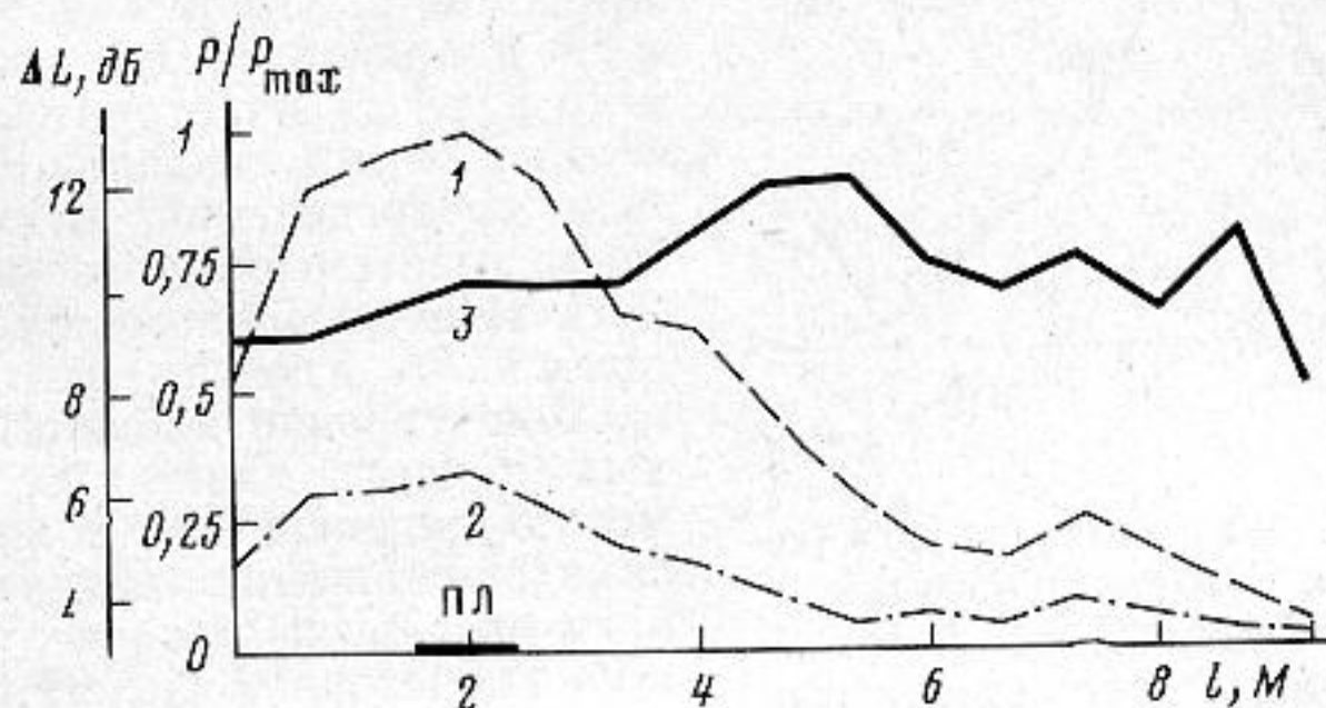
Фиг. 1. Зависимость амплитуды звукового давления, нормированного к максимальному значению, от расстояния l вдоль измерительной камеры на высоте 3 м. 1 — без компенсации, 2 — при компенсации, 3 — величина компенсации
