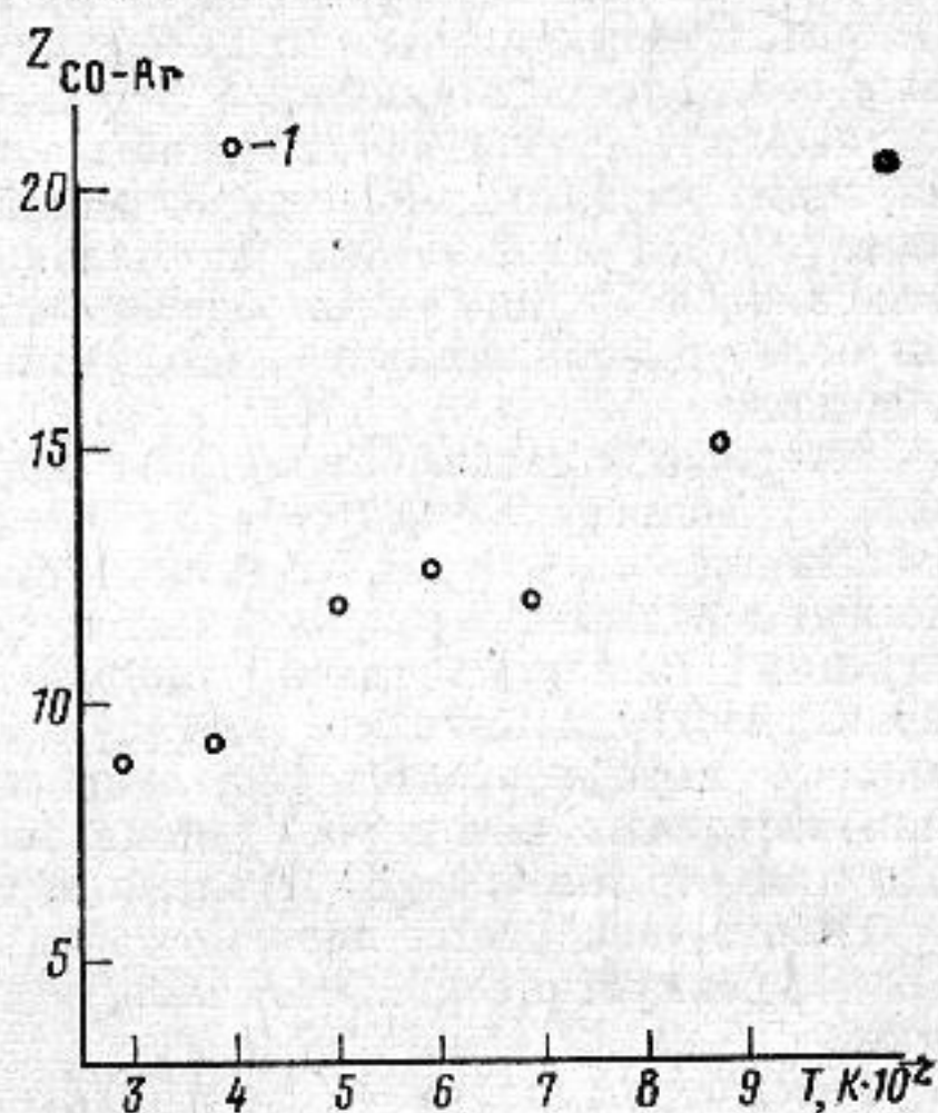
Температурная зависимость вращательных чисел столкновений Z_{\text{СО-Аг}}
