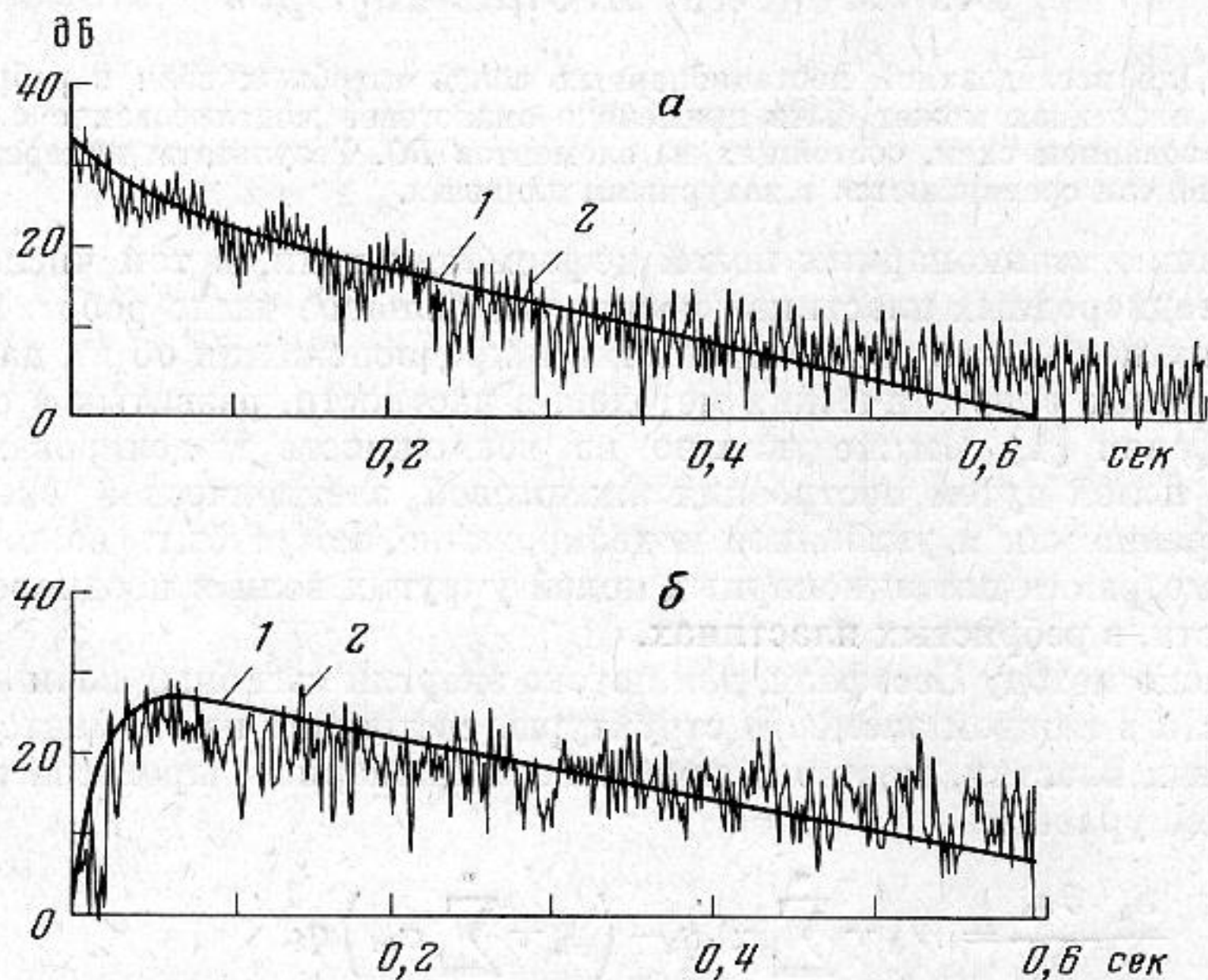
Фиг. 2. Зависимость от времени энергии изгибных волн в ребристой пластине и напряжения в ее электрической модели (а — в ячейке 1; б — в ячейке 6). 1 — модель; 2 — пластина
