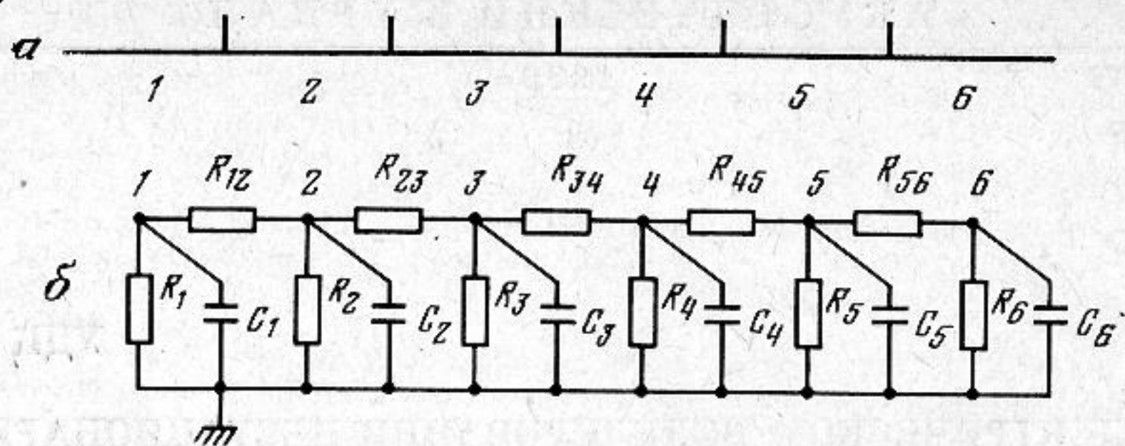
Фиг. 1. Конструкция ребристой пластины (а) и ее электрическая модель (б)
